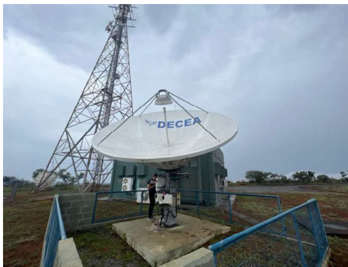
Imagem 11 – Fotos ilustrativas ATN-Br (VSAT)
